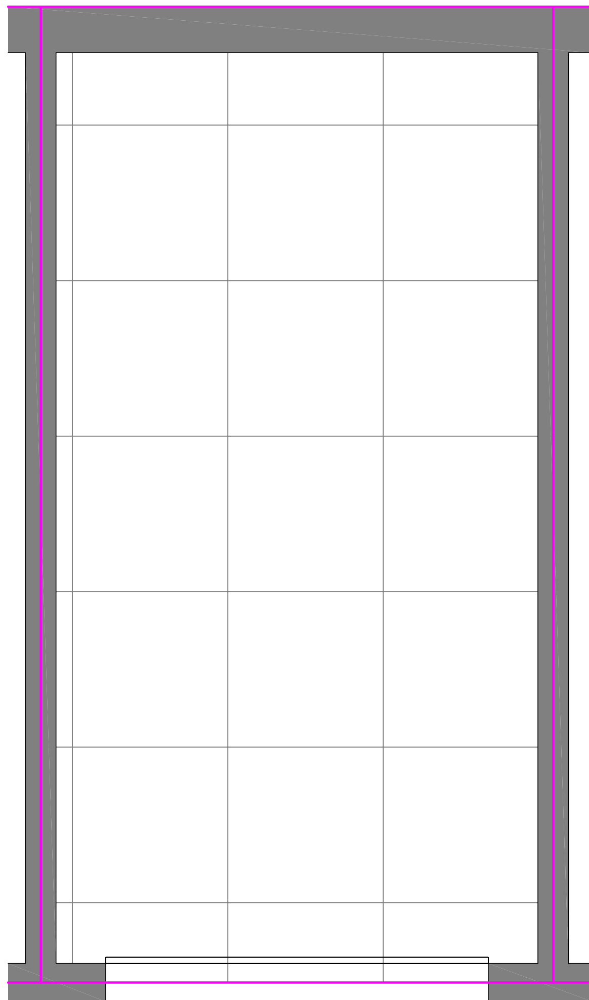
Pianta - Scala 1:25
